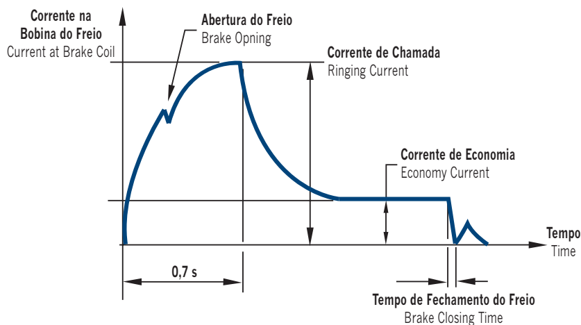
Características do Conversor C-4400-CE2 / Features of Converter C-4400-CE2
